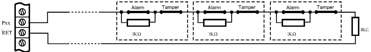
Rys 4. Podłączenie szeregowo urządzeń do linii parametrycznej
