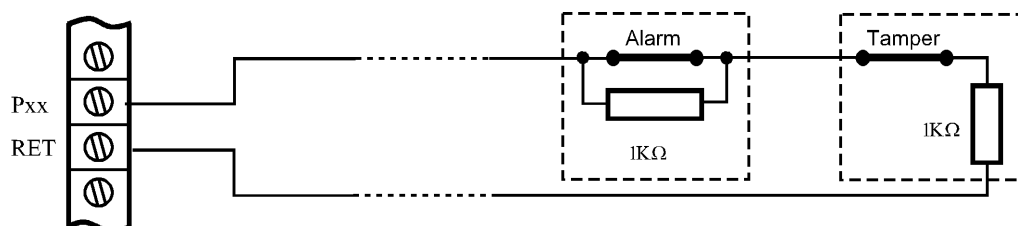
Rys 3. Podłączenie pojedynczego urządzenia do linii parametrycznej
